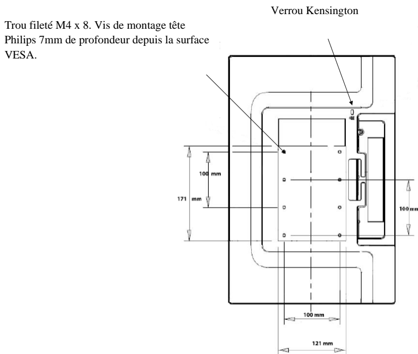
Vue arrière de l'écran en orientation portrait illustrée ci-dessus
