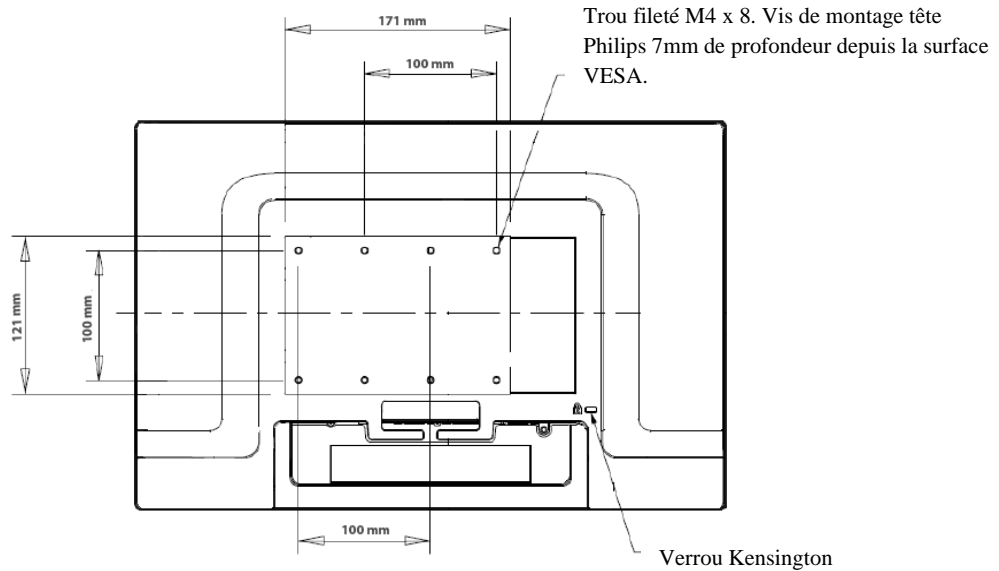
Vue arrière de l'écran en orientation paysage illustrée ci-dessus
